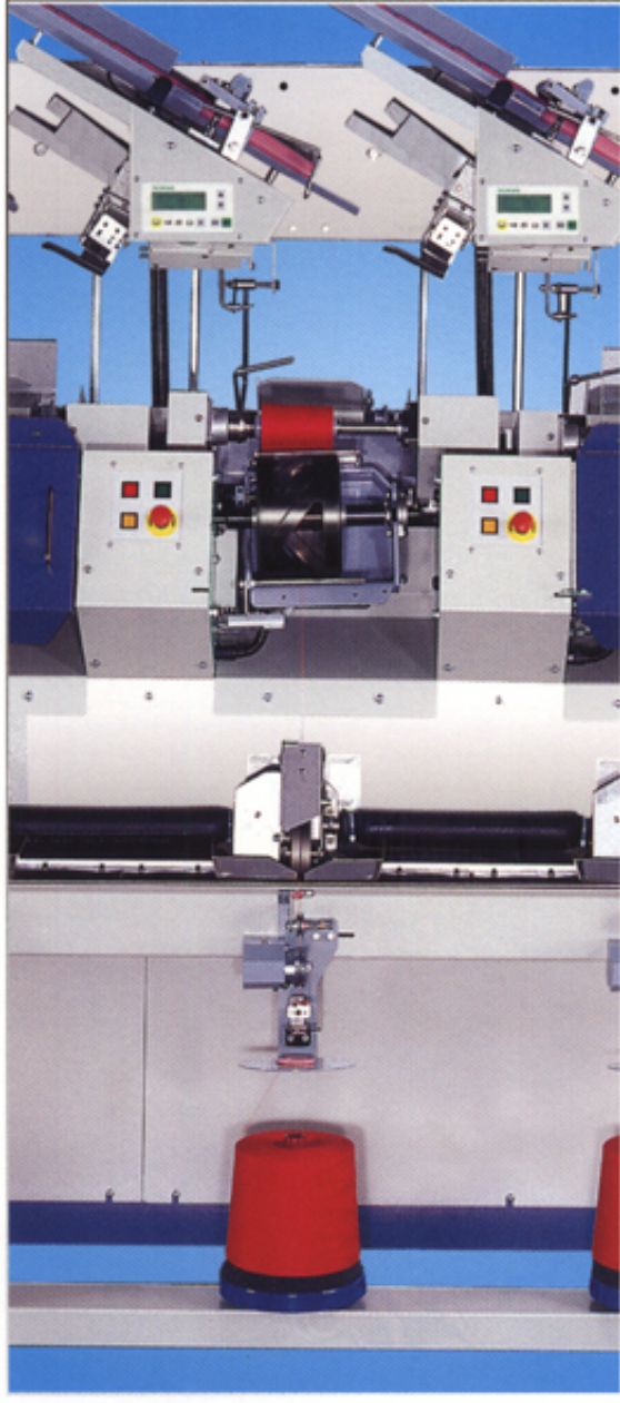
TN-35A 全自動高速繞線機-H型管
