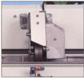
可設定目跟隨線速之上油裝置
