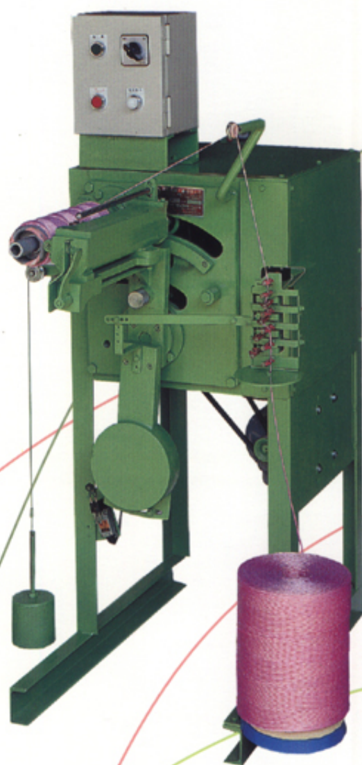
捲線機 Cross Cone Winder
